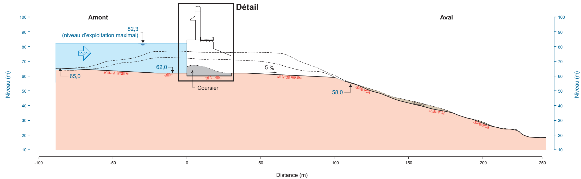
Évacuateur de crues – Profil longitudinal A
