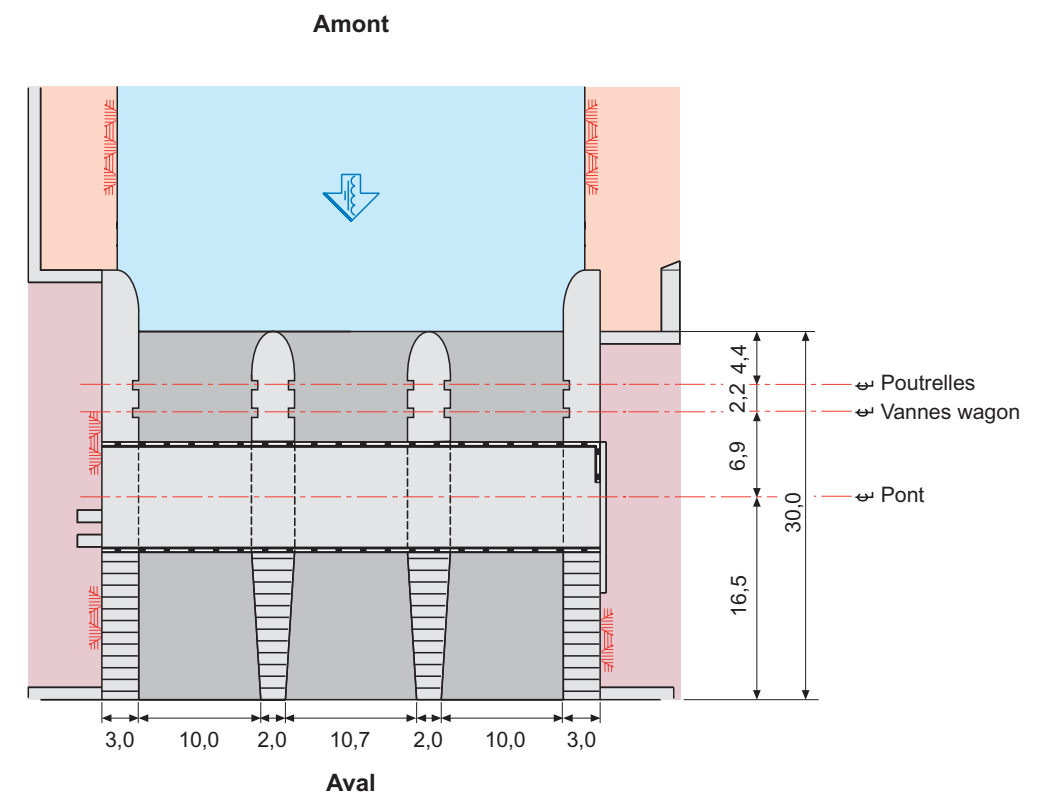
Évacuateur de crues – Vue en plan
