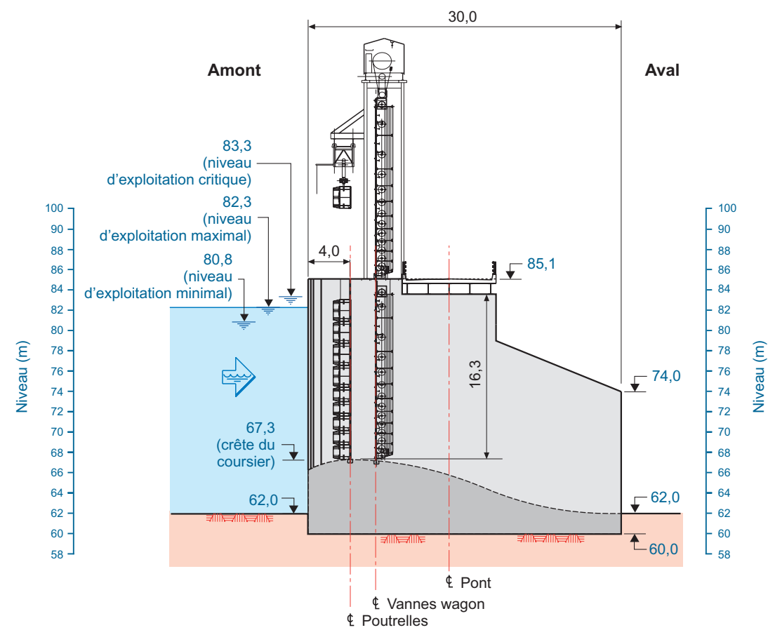
Évacuateur de crues – Détail
